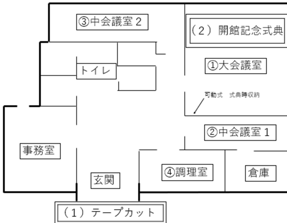
新小来川公民館レイアウト
