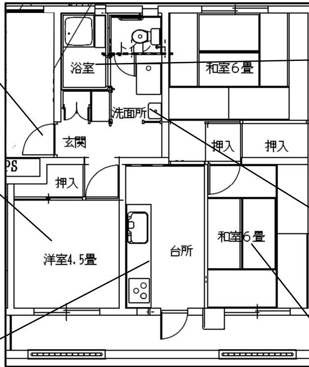
3DK
