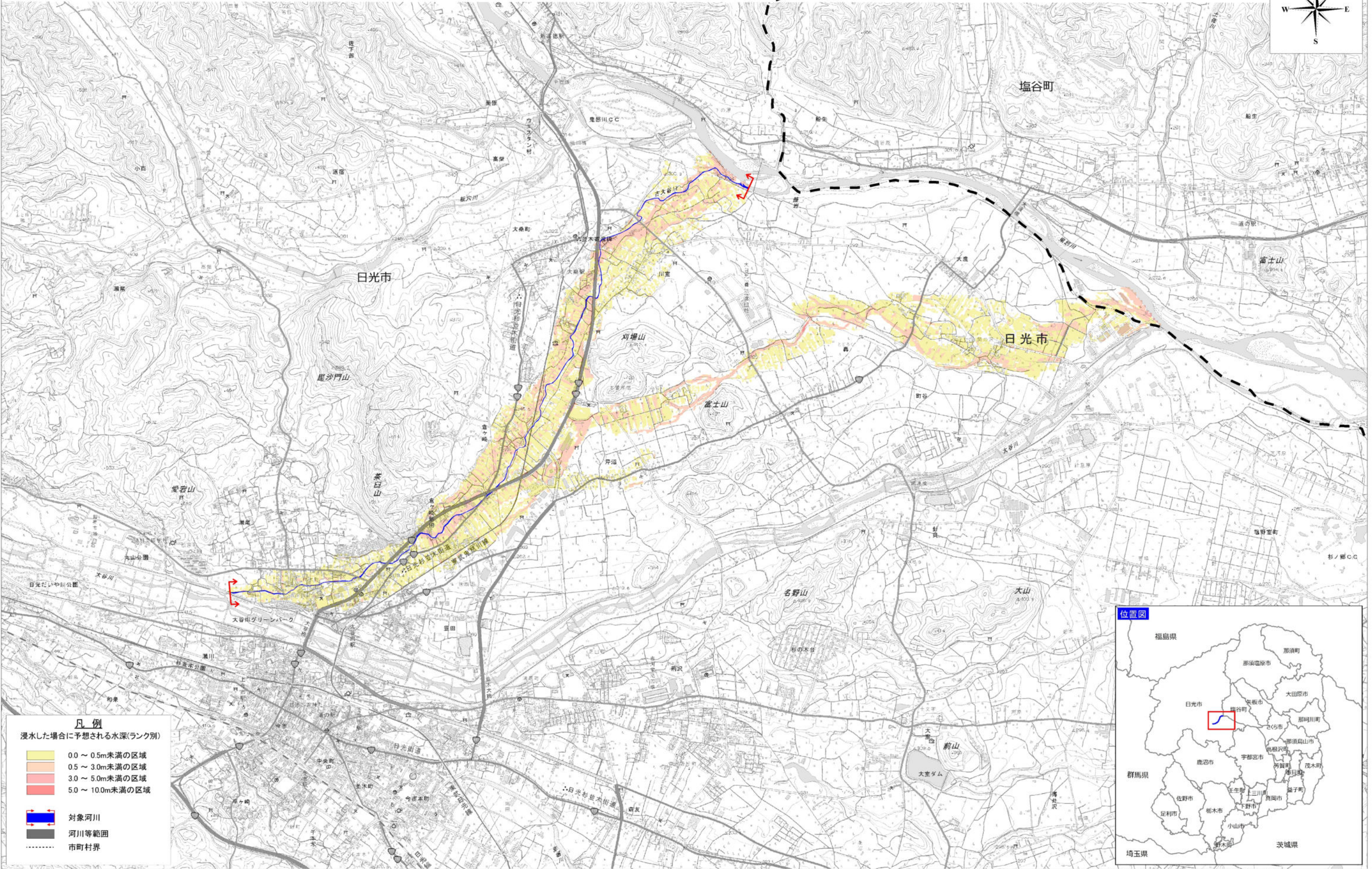
利根川水系古大谷川洪水浸水想定区域図 想定最大規模（全体図）
