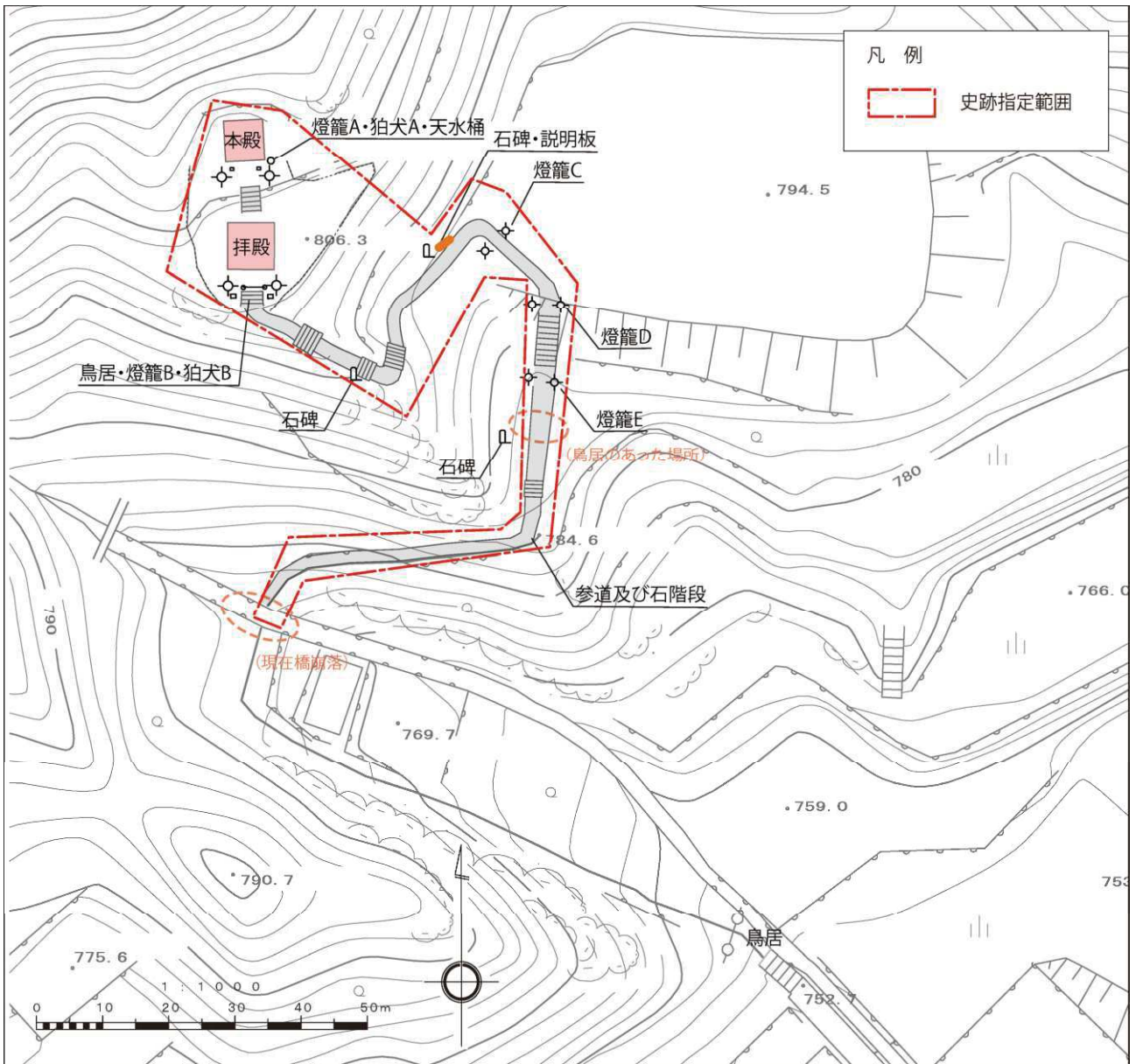
图 2-38 構成要素図 (本山鉦山神社跡)
