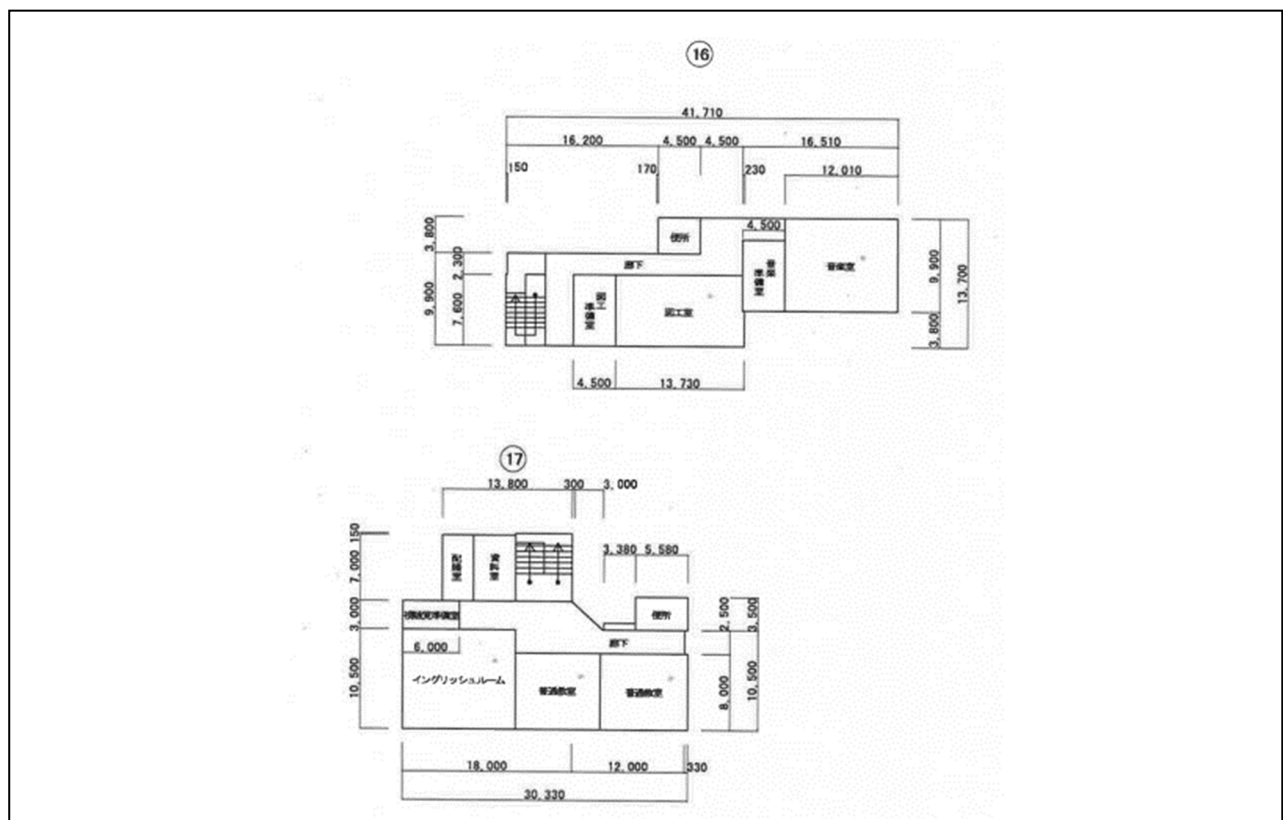
平面図 (3階)
